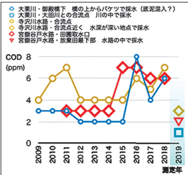
図1 由木地区環境市民会議によるCOD測定値の年次推移
